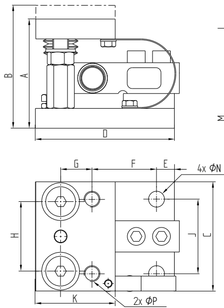
STABIFLEX-SK EVO ohne Stabilisator
